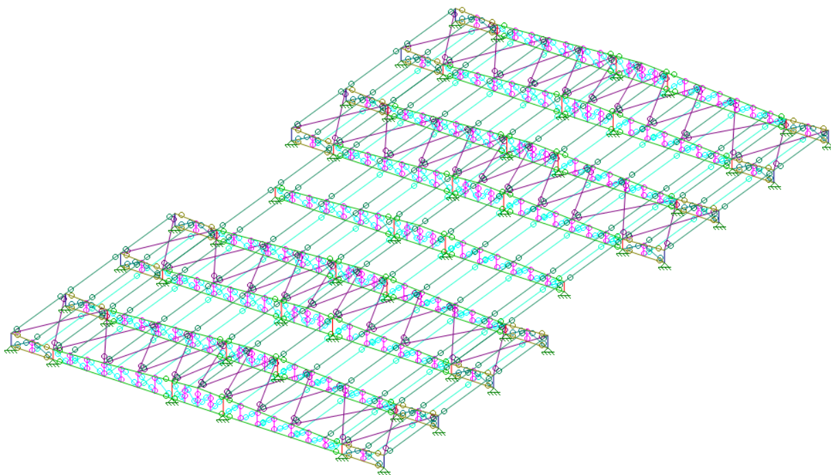
FIGURA 5 - VISTA 3D COBERTURA BLOCO B
