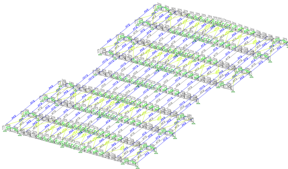
FIGURA 14 - MODELO UNIFILAR DIMENSIONADO - COBERTURA BLOCO B
