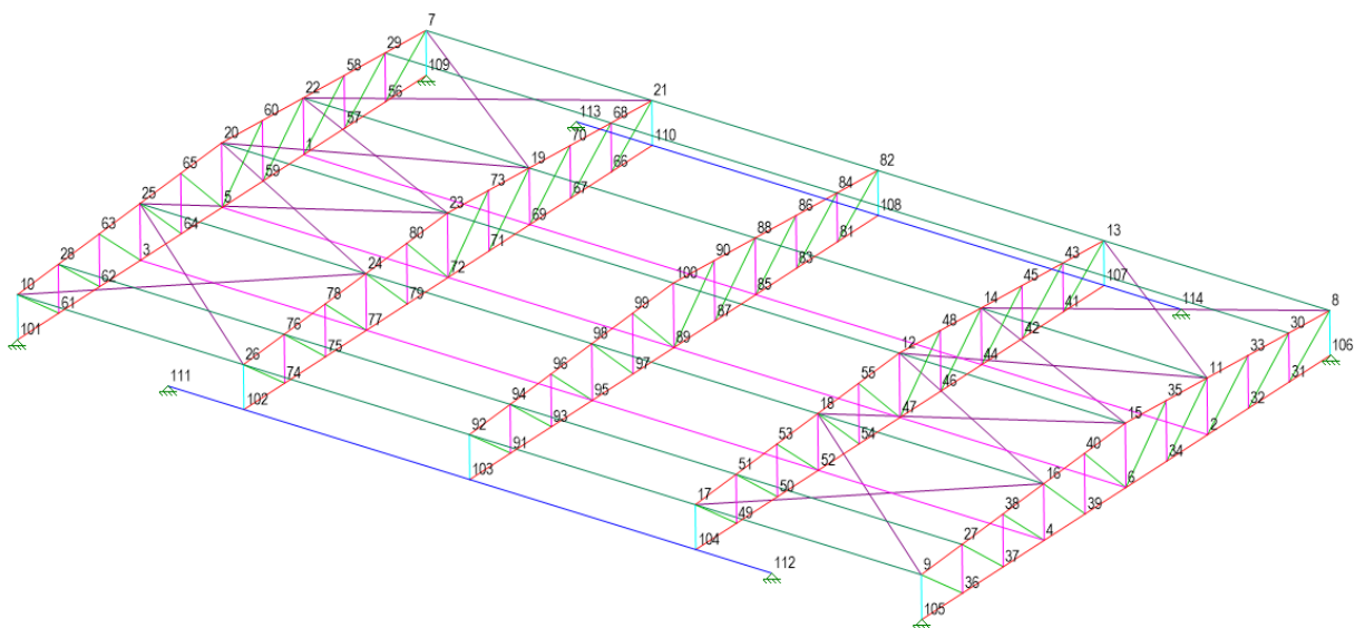
FIGURA 7 - NÓS DA COBERTURA BLOCO LIGAÇÃO
