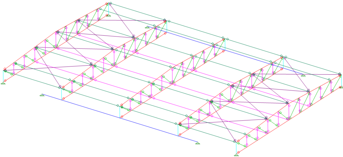
FIGURA 4 - VISTA 3D COBERTURA BLOCO LIGAÇÃO
