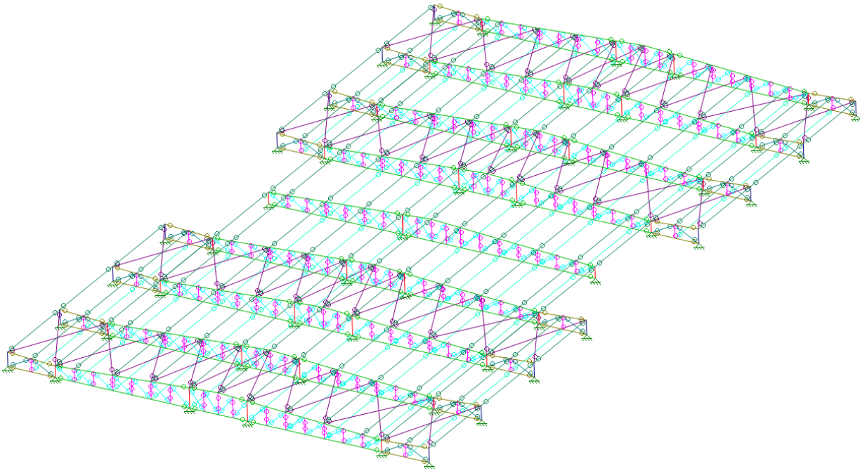
FIGURA 3 - VISTA 3D COBERTURA BLOCO A
