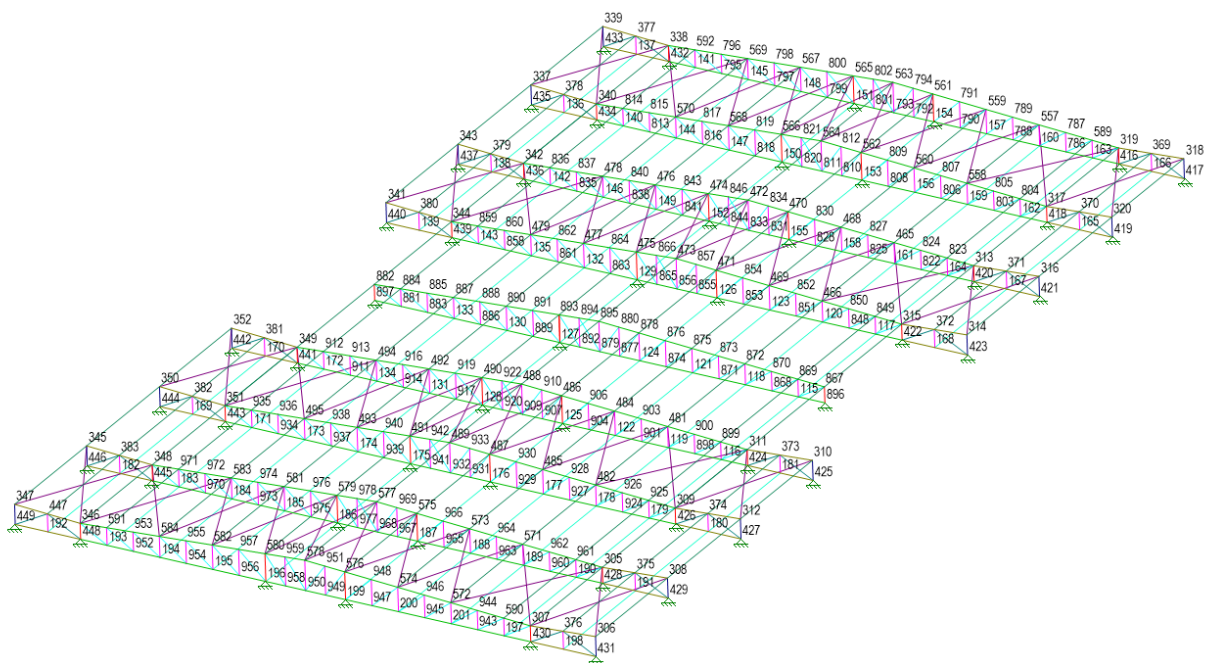
FIGURA 6 - NÓS DA COBERTURA BLOCO A
