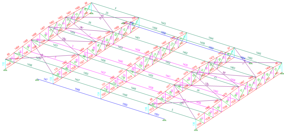
FIGURA 10 - BARRAS DA COBERTURA BLOCO LIGAÇÃO
