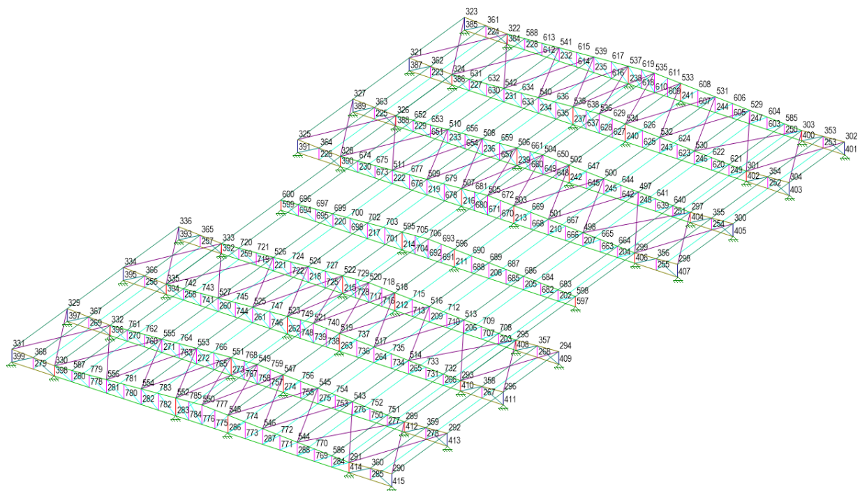
FIGURA 8 - NÓS DA COBERTURA BLOCO B
