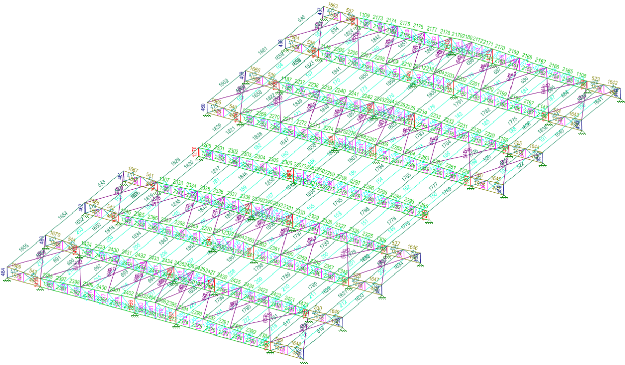
FIGURA 9 - BARRAS DA COBERTURA BLOCO A
