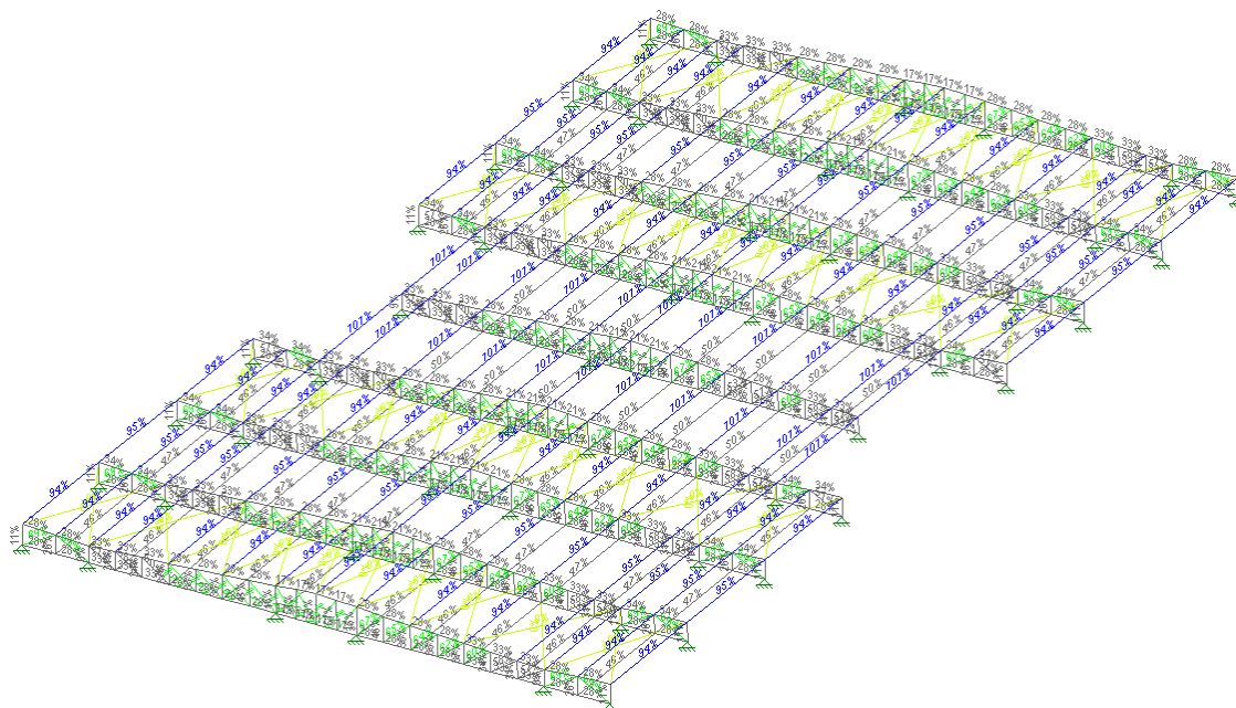
FIGURA 12 - MODELO UNIFILAR DIMENSIONADO - COBERTURA BLOCO A
