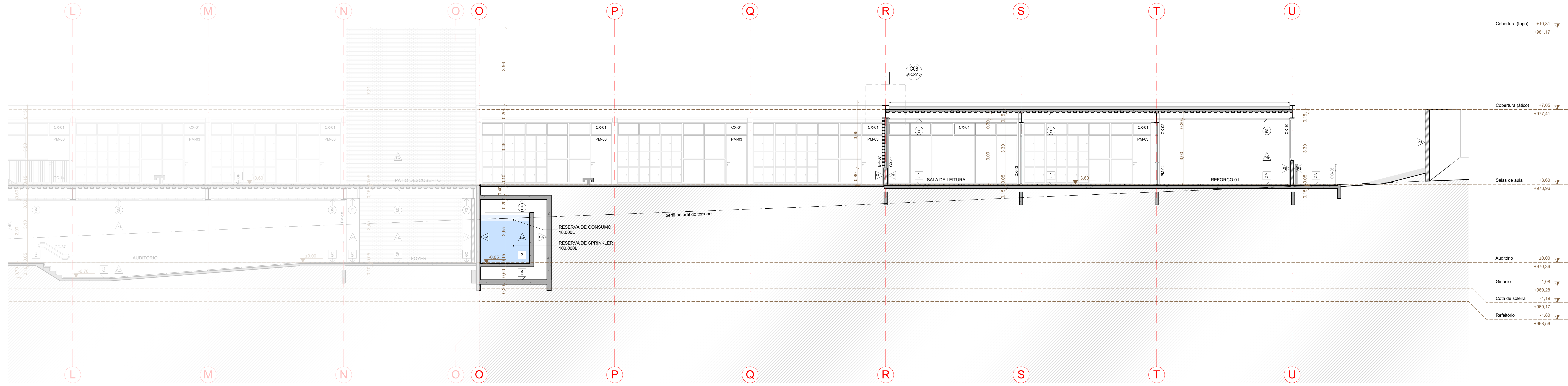
CORTE BB - TRECHO C ESCALA 1/75
