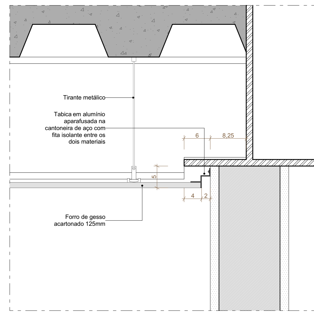
F05 DETALHE FORRO ESCALA 1:5
