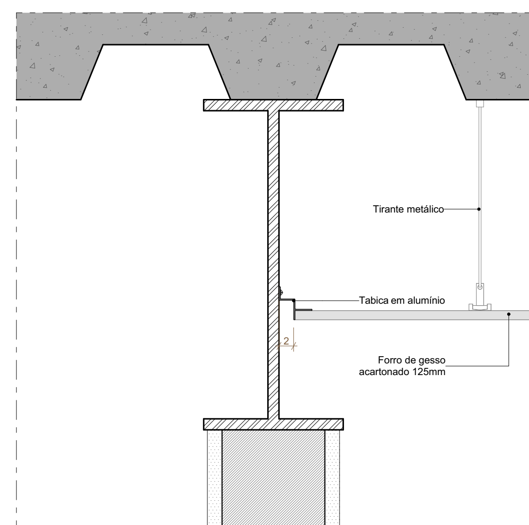
F22 DETALHE FORRO ESCALA 1:5
