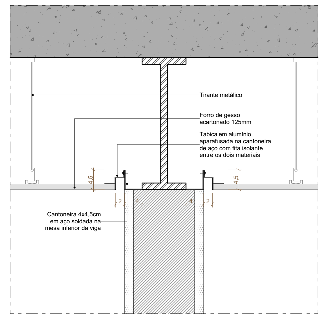
F08 DETALHE FORRO ESCALA 1:5
