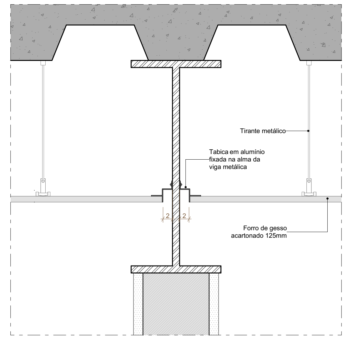
F02 DETALHE FORRO ESCALA 1:5
