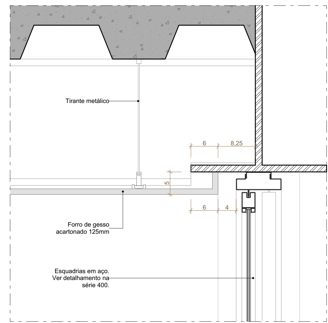
F06 DETALHE FORRO ESCALA 1:5
