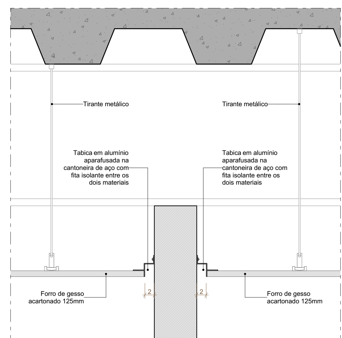
F24 DETALHE FORRO ESCALA 1:5
