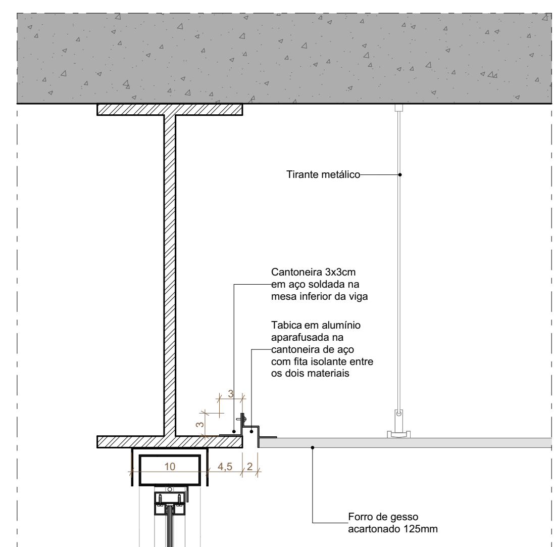
F11 DETALHE FORRO ESCALA 1:5
