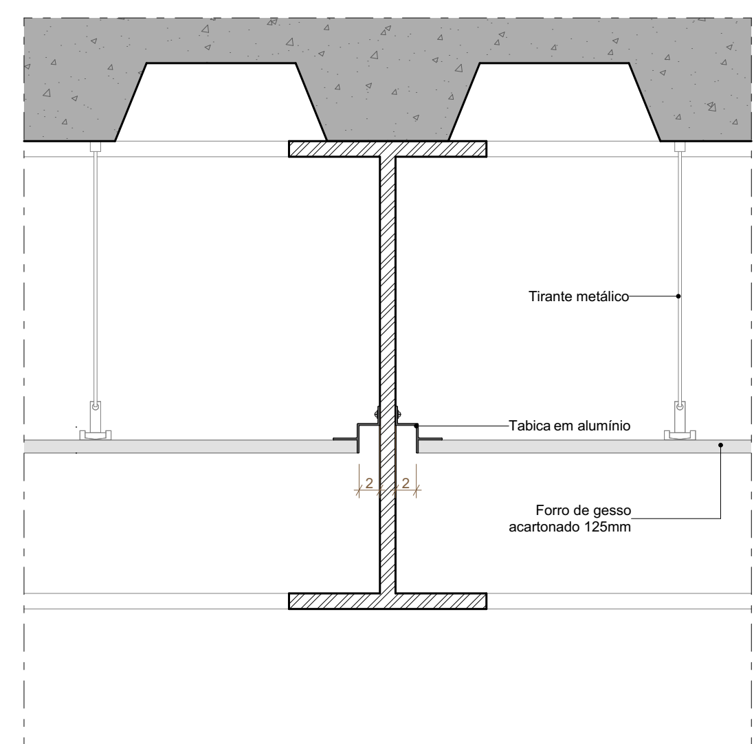
F12 DETALHE FORRO ESCALA 1:5
