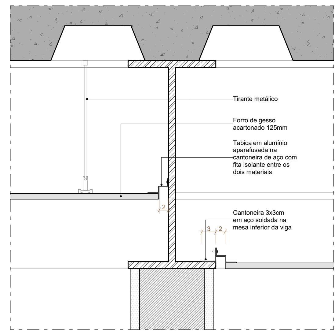
F07 DETALHE FORRO ESCALA 1:5
