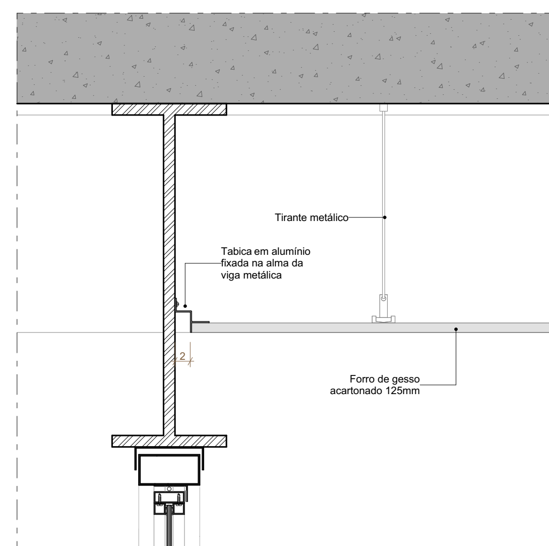
F09 DETALHE FORRO ESCALA 1:5
