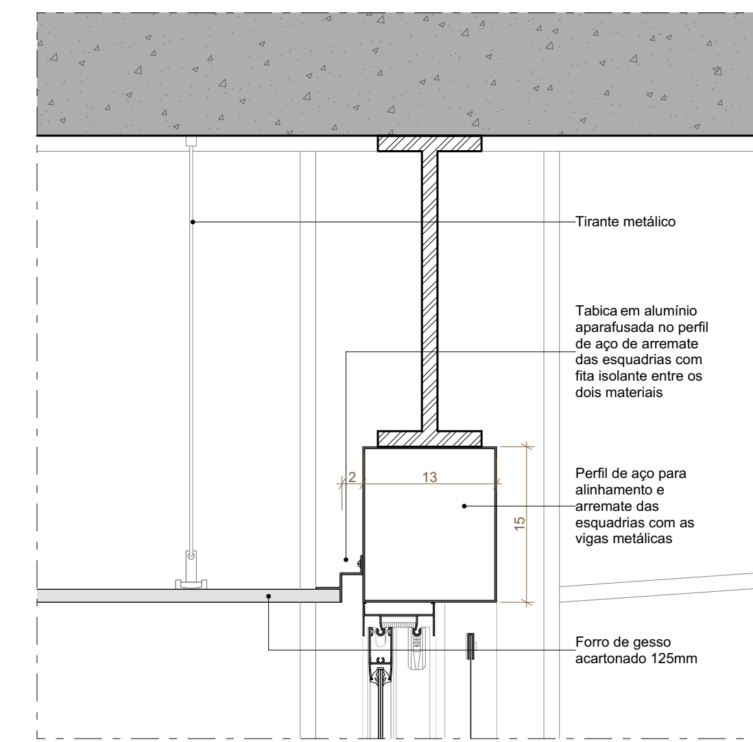
F27 DETALHE FORRO ESCALA 1:5
