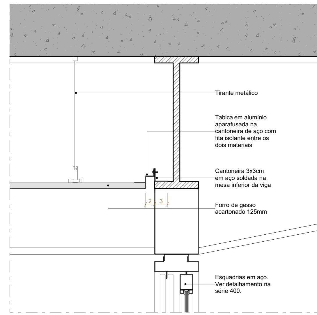
F01 DETALHE FORRO ESCALA 1:5
