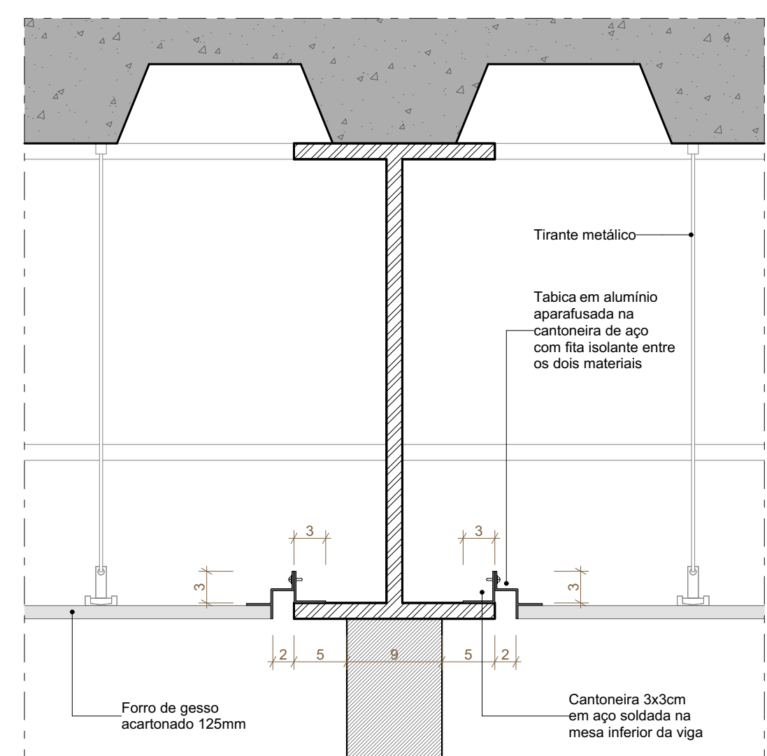
F25 DETALHE FORRO ESCALA 1:5
