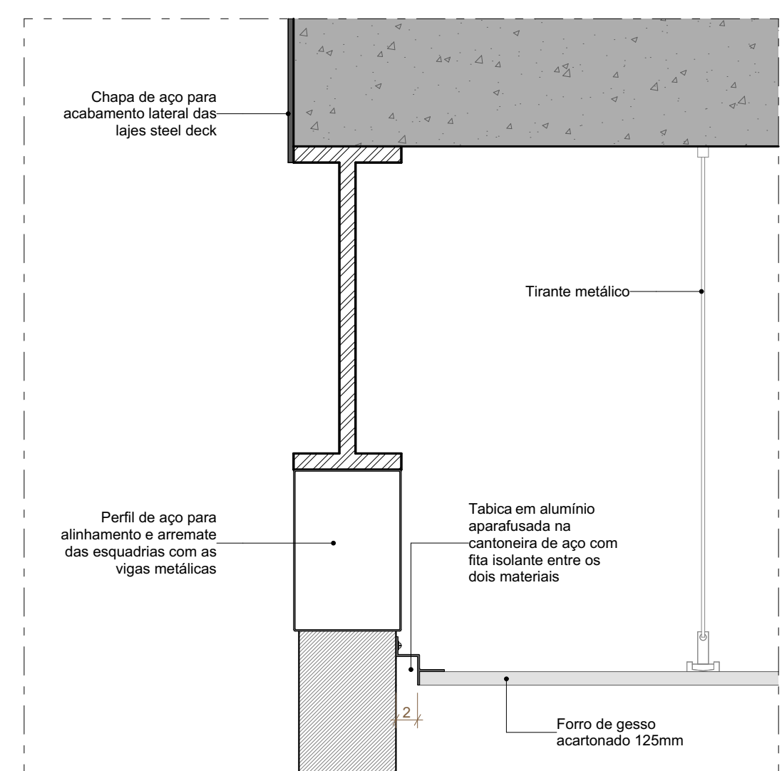
F23 DETALHE FORRO ESCALA 1:5
