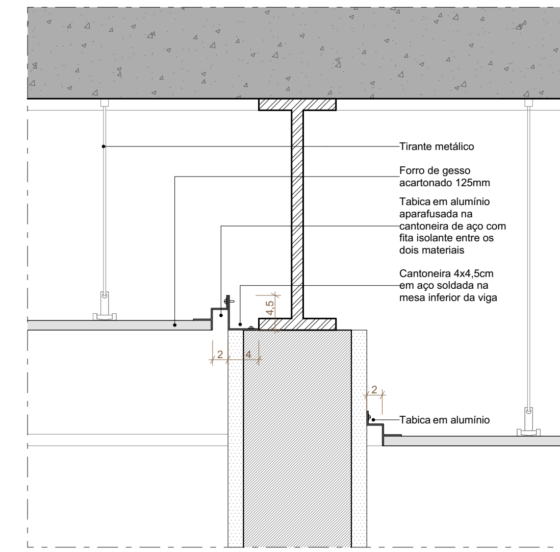
F26 DETALHE FORRO ESCALA 1:5
