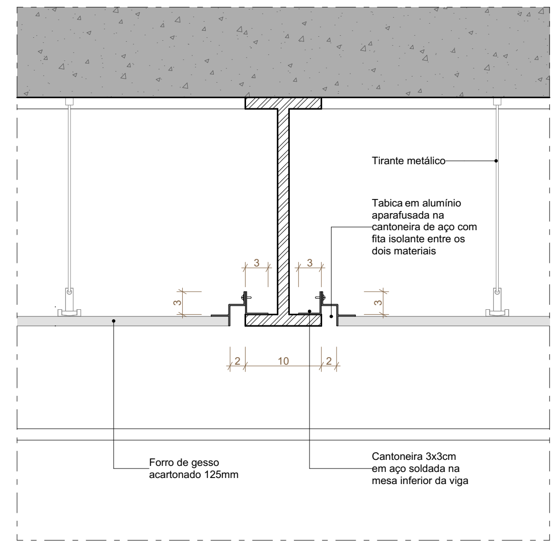
F03 DETALHE FORRO ESCALA 1:5
