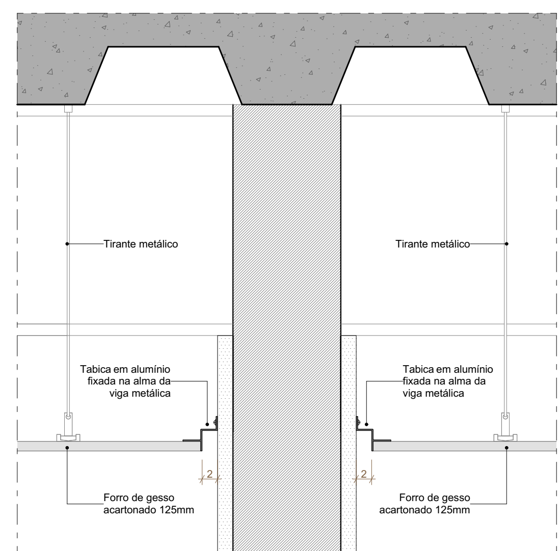
F10 DETALHE FORRO ESCALA 1:5
