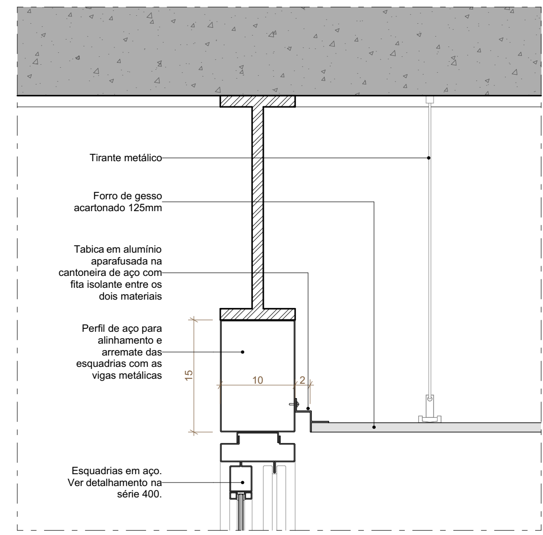
F04 DETALHE FORRO ESCALA 1:5
