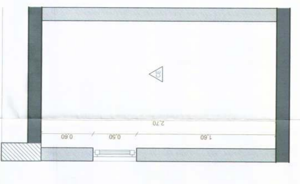
E14.5 WC Guarita Escala: 1:25
